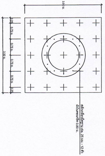
แบบขยายฐานรากหลอดสูง (แบบเสาเข็ม) ขนาดพื้นที่ 1 : 50
